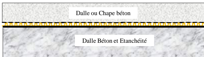
Pose ALVEODRAIN F et joints radiaux
